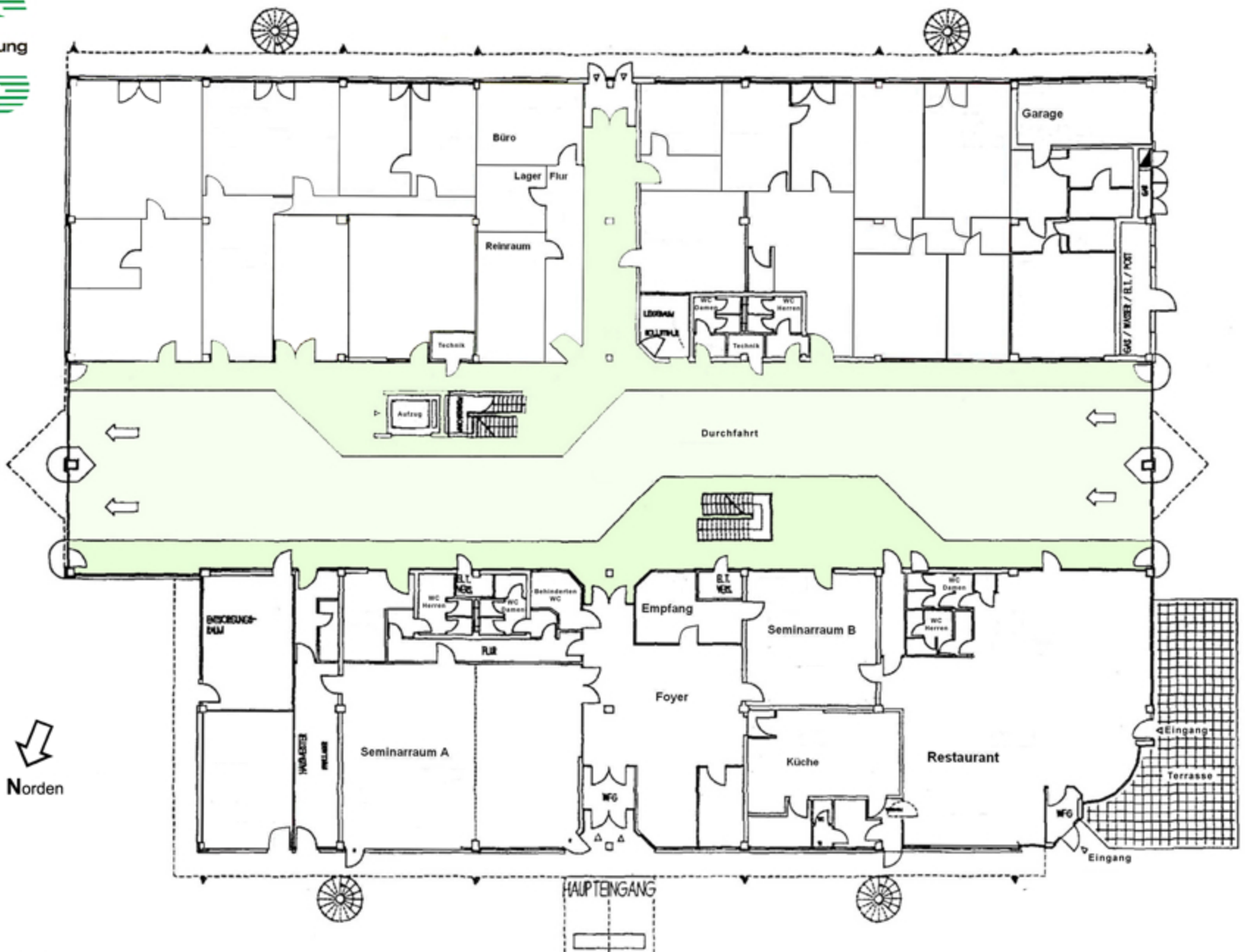
Grundriss Erdgeschoss Raumaufteilung der Nutzungseinheiten
